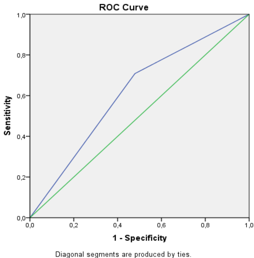
16. ábra. A „MEDIANKAT” változó ROC görbéje
