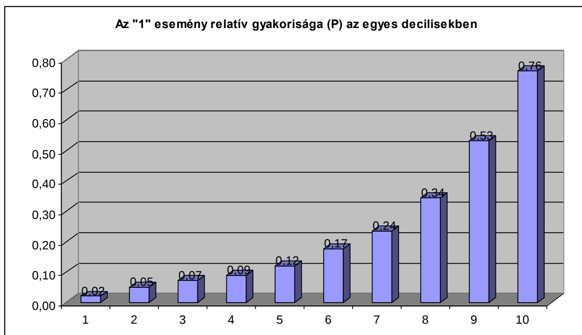
19. ábra. Relatív gyakoriságok az egyes decilisekben
