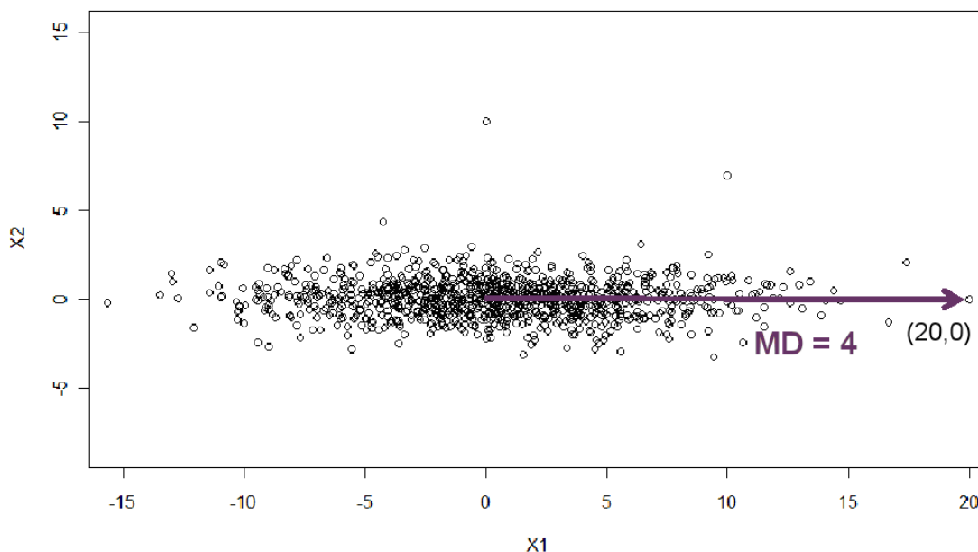
9. ábra. Mahalanobis távolság 4
