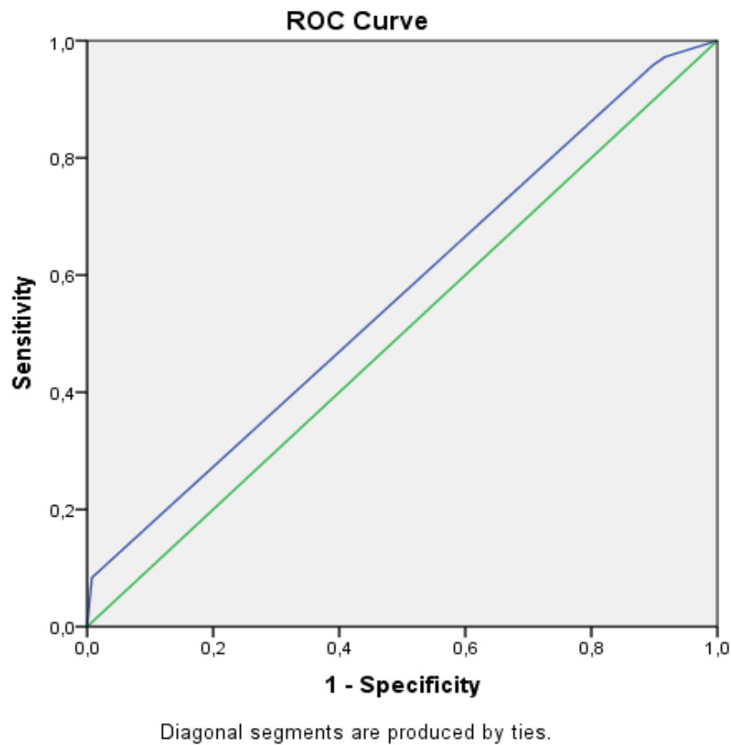
15. ábra. A „SCALEKAT” változó ROC görbéje
