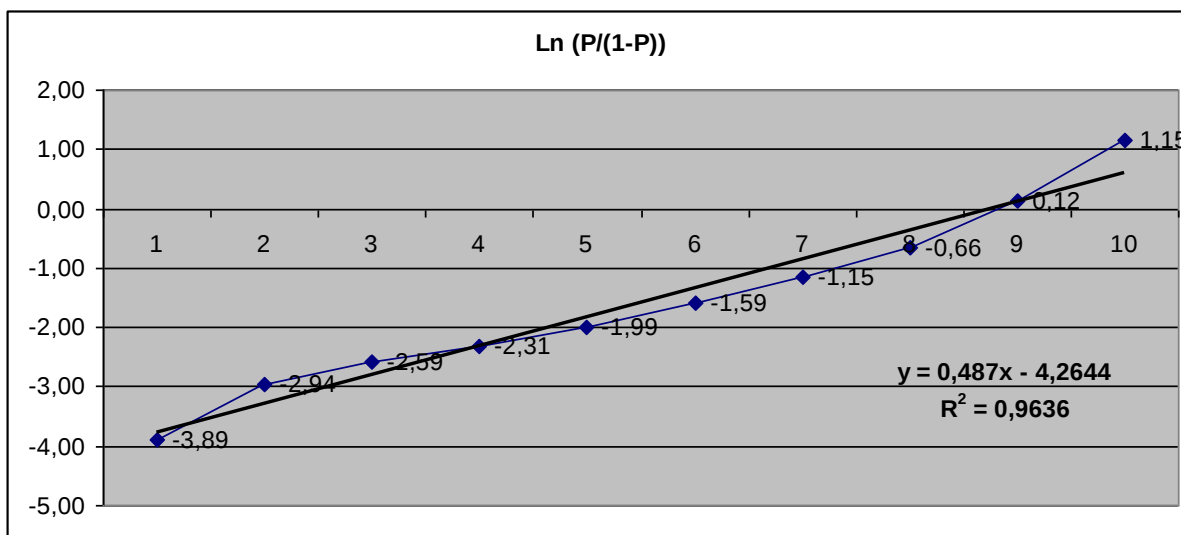
20. ábra. Regressziós egyenes illesztése
