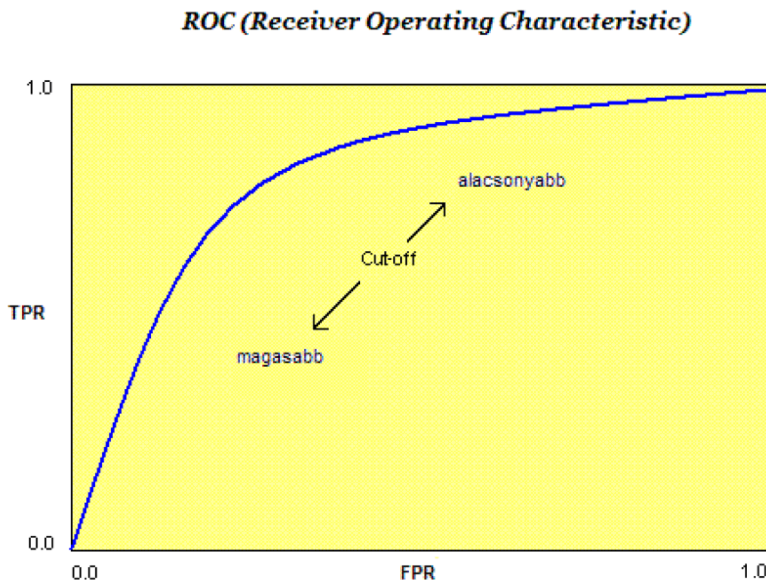
3. ábra. ROC görbe
