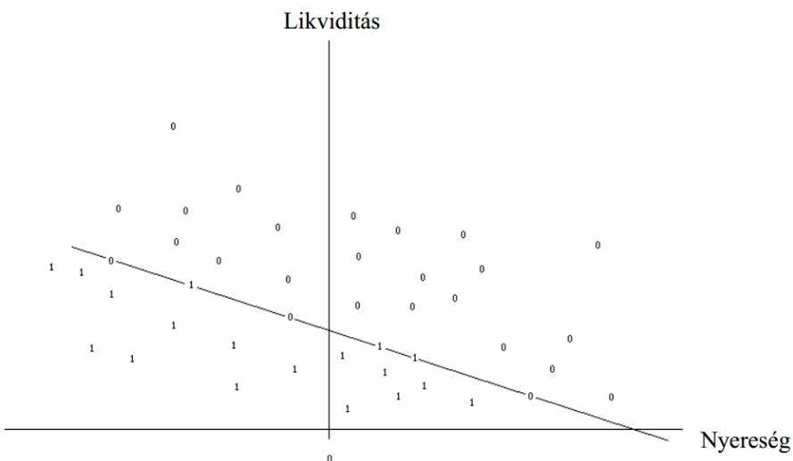
Kváziszeperált megfigyelések két magyarázóváltozó síkjában
