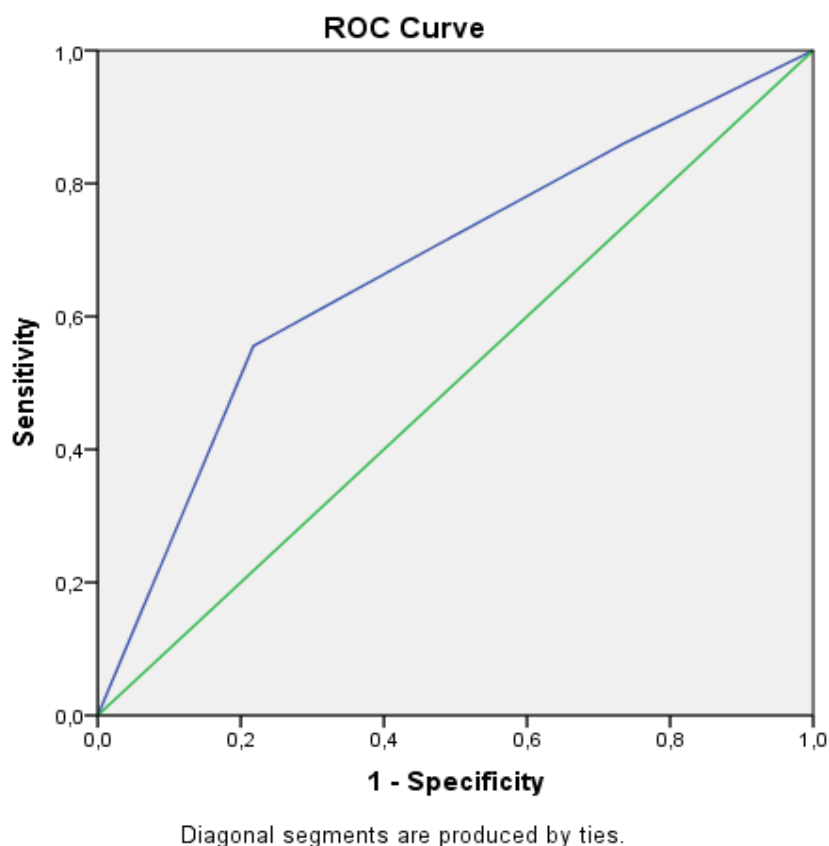
14. ábra. A „Q123KAT” változó ROC görbéje
