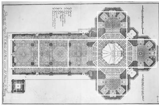
8. kép. A Santa Maria del Fiore alaprajza Warren két mérési alapegységének feltüntetésével
