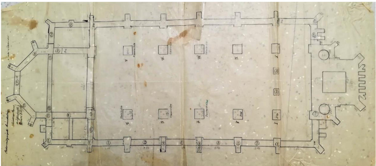
15. Az 1911-ben véglegesített templom alaprajz - GyFLSzGyl,712/e, 18, 1. cs.
