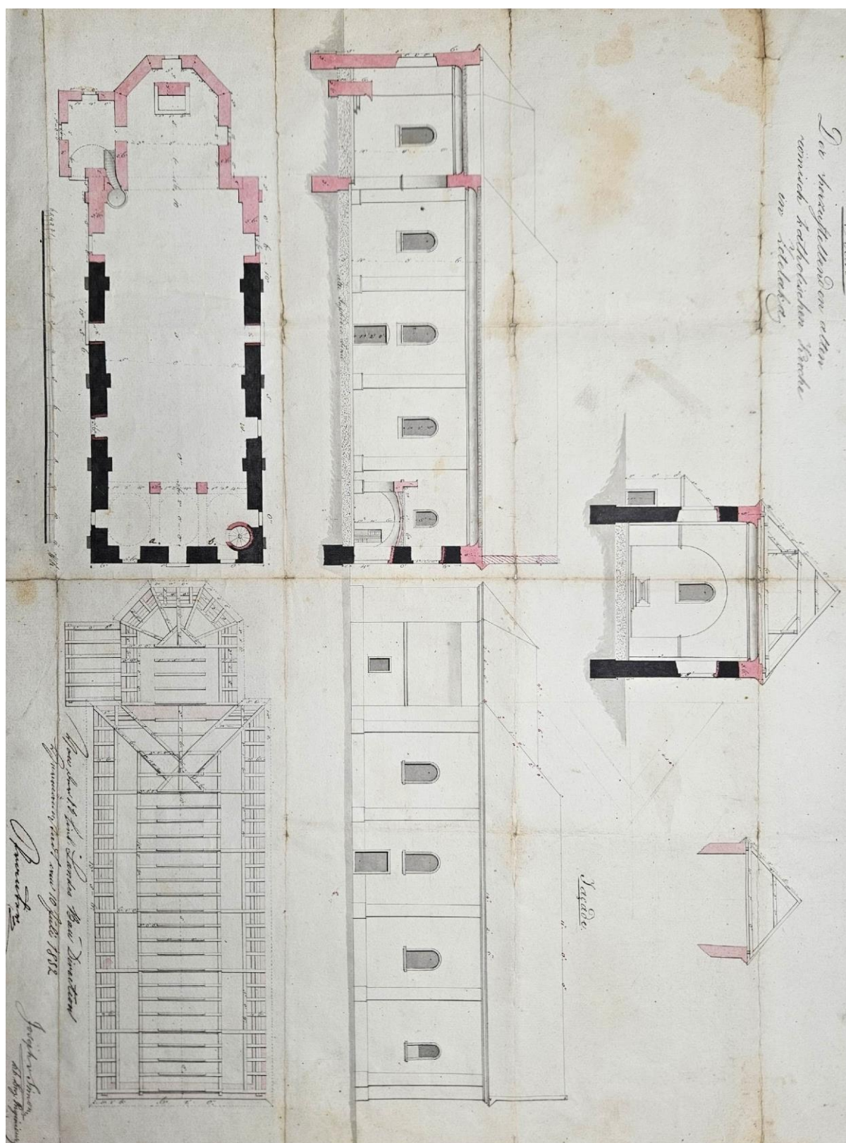
1. Simó József 1852-ben készült templomjavítási terve - GyFLSzGyl,712/e, 18, 1. cs.
