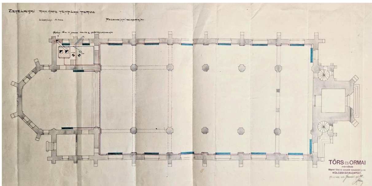
17. Törs és Ormai cég által készített központifűtés tervrajz - GyFLSzGyl,712/e, 19, 6. cs.
