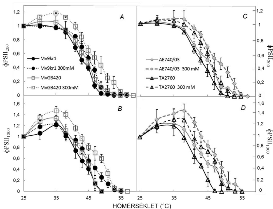
22. ábra. A PSII effektív kvantumhatásfokának ( \Phi_{PSII} ) egyre normalizált értékeinek hőmérsékletfüggése a kontroll (folytonos vonal) és a 300 mM NaCl kezelt (szaggatott vonal) búza (Mv9kr1) és Ae. umbellulata (MvGB 420) vonalakban 200 \mu E\ m^{-2}s^{-1} (A) és 1000 \mu E\ m^{-2}s^{-1} fényintenzitáson (B), valamint az Ae. umbellulata (AE740/03) és Ae. comosa (TA 2760) vonalakban 200 \mu E\ m^{-2}s^{-1} (C) és 1000 \mu E\ m^{-2}s^{-1} fényintenzitáson (D). A feltüntetett értékek a kezelésenkénti öt ismétlés átlagait mutatják a standard hibával
