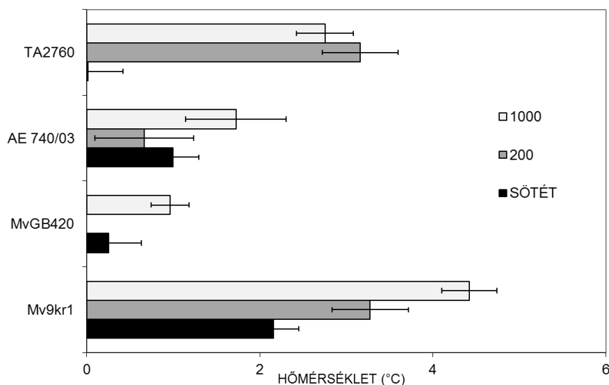
19. ábra. A 10 napos vízhiány hatása a búza (Mv9kr1), az Aegilops umbellulata vonalak (MvGB 420, AE 740/03) és az Aegilops comosa vonal (TA 2760) fenotípusos plaszticitására (Tc 1 -Tc 0 ) sötétben, 200 μE m -2 s -1 (200) és 1000 μE m -2 s -1 (1000) fényintenzitáson a kontroll és a 10 napos szárazságkezelésnél regisztrált Tc pontok alapján. A feltüntetett értékek a kezelésenkénti öt ismétlés átlagait mutatják a standard hibával
