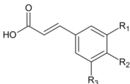
Hidroxi-fahéjsavak
