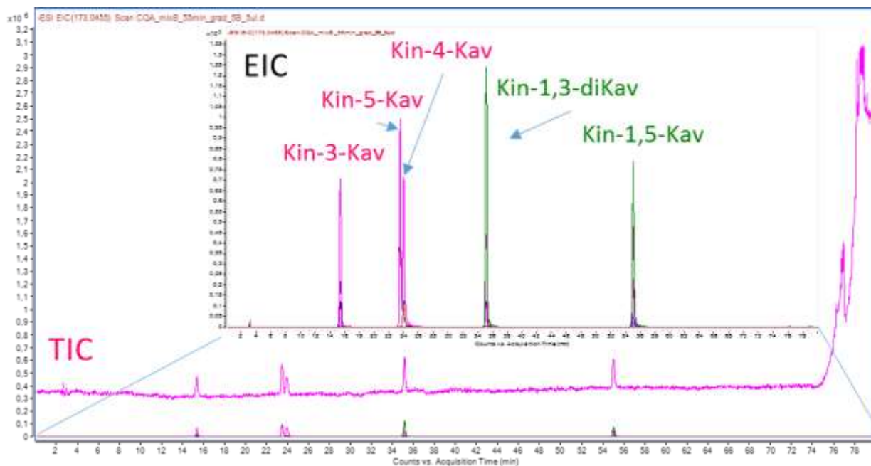
13. ábra: Kinasav-O-hidroxi-fahéjsav észter referencia oldat egymásra lapolt ionkromatogramjai.
