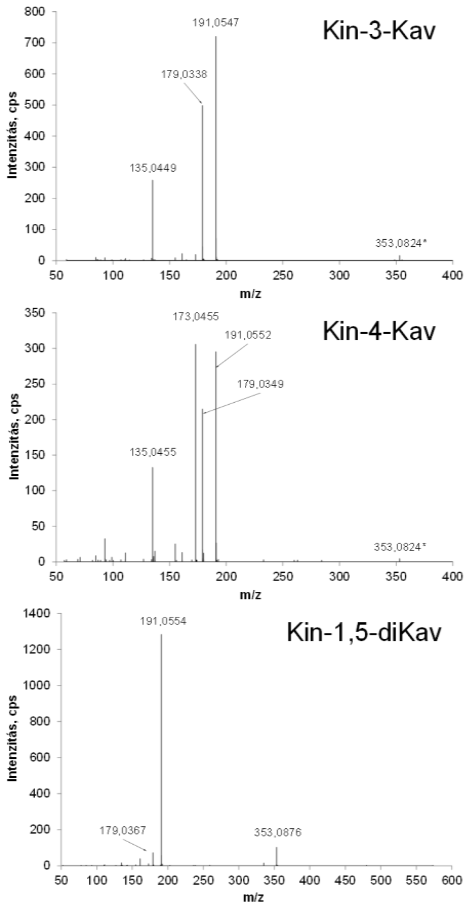
15. ábra: Kinasav- O -hidroxi-fahéjsav észterek MS/MS fragmentációs spektruma.
