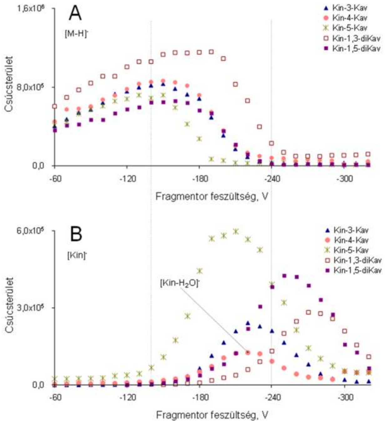
16. ábra: Forrásban történő CID fragmentáció optimalás fragmentor feszültség segítségével.
