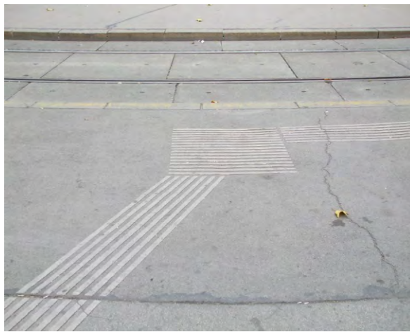
370. szinkontraszt az útpályával; csak vezetőelemek használata
