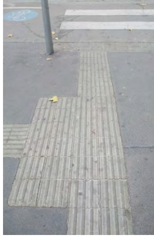
366-368. csekély szinkontrasztú TWSI Bécsben; figyelmeztetéskeresztbe fordított vezetőelemekkel
