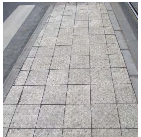
292-293. ha a vezetősáv átkelő tengelyével való párhuzamos kialakítása nem lehetséges, akkor is tartson az átkelőhelyen belül
