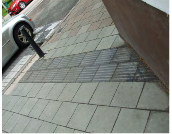
328-330. a figyelmeztetősáv az útburkolati jelekkel megegyező színű és szélességű; a vezetősáv csupán enyhe szinkontrasztot mutat
