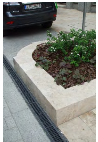
147-150. a gyalogos közlekedési tengelybe eső természetes vezetősávok (homlokzatok, növénykazetták, zöldsávok, szegélyek) tisztán tartása alapvető követelmény - a belógó növényzet, a jelölés nélkül, nem következetesen elhelyezett tereptárgyak akadályt jelentenek
