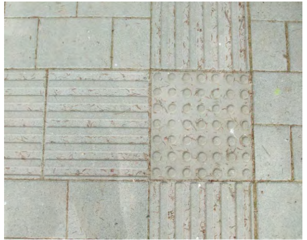
732-734. taktilis jelzés bemutatóközpont térköburkolatában: épületek környezetében a szilárd burkolat használata is indokolt lehet
