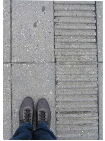
196-198. a térszervezés indokolta burkolatváltások egyben a különböző forgalmi sávok, kültéri funkciók elkülönítésére is alkalmasak
