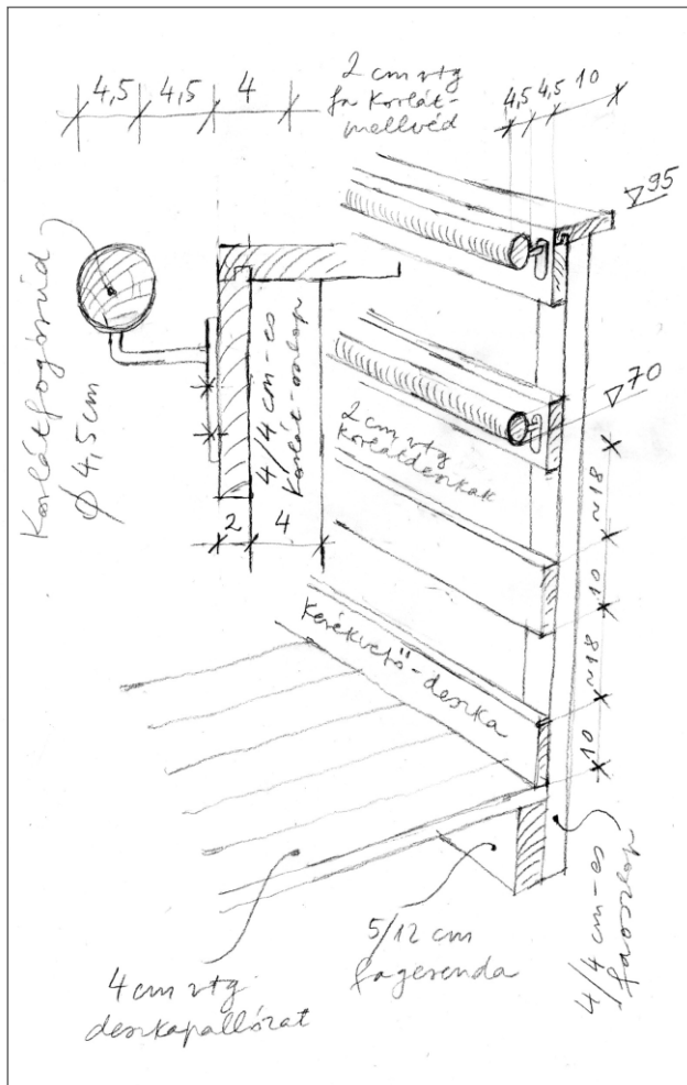
846. tervezett akadálymentes korlát a tábori pallórendszerhez
