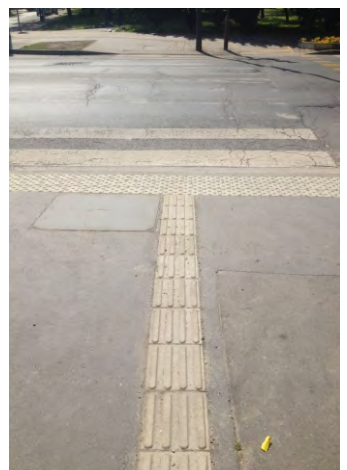
261-262. a fehér jelzés könnyen koszolódik, ezért a kontraszt megőrzése érdekében tisztítani kell
