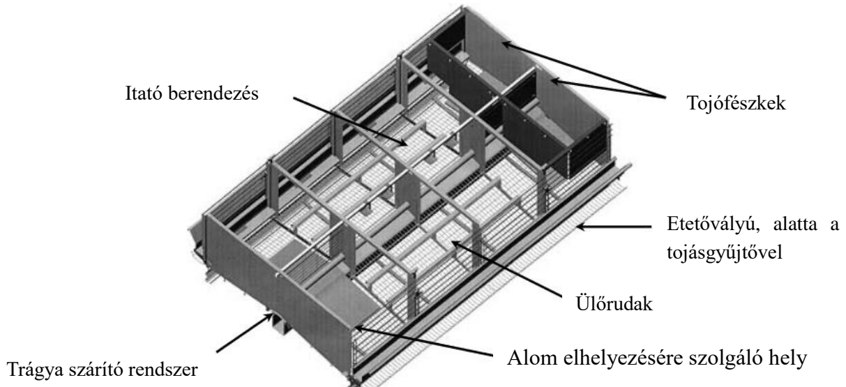
2. ábra: Nagycsoportos feljavított ketrec ("large furnished cage") berendezése
