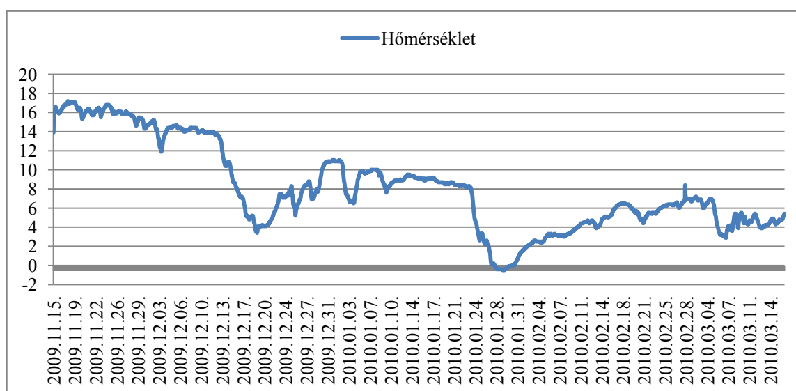
19. ábra: A 2009/2010. vizsgálati évben végzett teletetési kísérlet során mért hőmérsékleti adatok 1 m mélyen Celsius fokban
