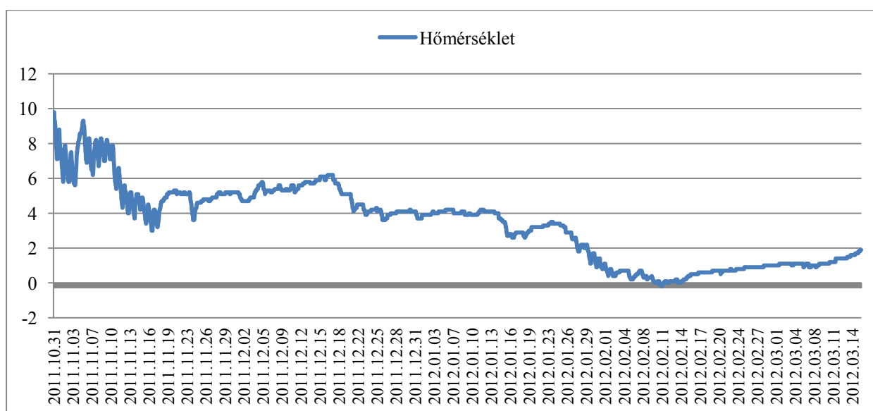
24. ábra: A 2011/2012. vizsgálati évben végzett telettétési kísérlet során mért hőmérsékleti adatok 1 m mélyen Celsius fokban
